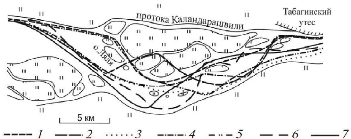
Рисунок 3.14 — Изменения положения судовой ходы в «разбое» Рассолода: 1 — 1934 г.; 2 — 1951 г.; 3 — 1972 г.; 4 — 1982 г.; 5 — 2000 г.; 6 — 2010 г.; 7 — 2017 г.). [Чалов, Завадский, и др., 2019].
