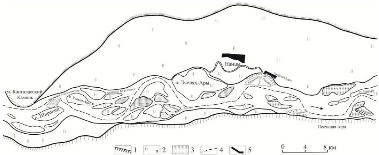
Рисунок 3.18 — Общая схема узлов разветвления на р. Лене ниже Кангаласского мыса: 1 — коренные борта долины; 2 — высокая и низкая пойма; 3 — прирусловые отмели, осередки; 4 — положение судового хода; 5 — населенные пункты.
