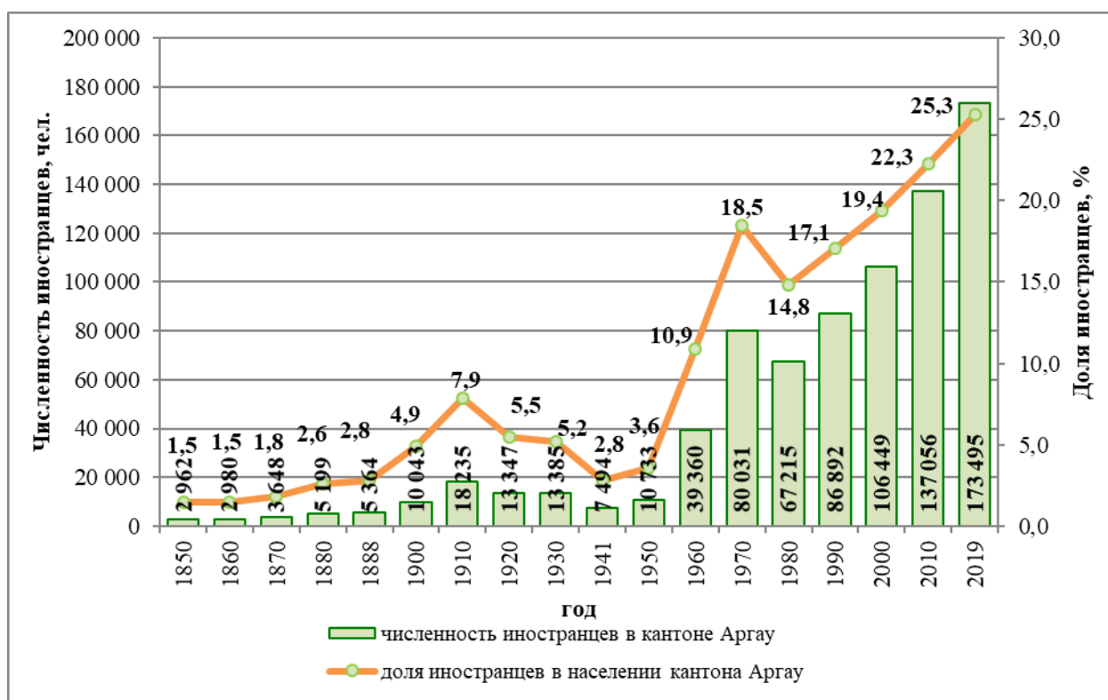
Рис. 7.2. Численность и доля иностранных граждан в населении кантона Аргау, 1850–2019 гг.
