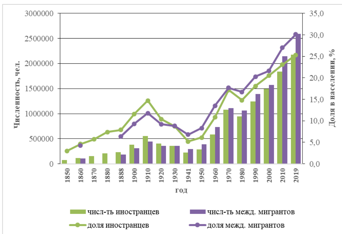
Рис. 1. Швейцария: численность и доля в населении страны международных мигрантов и иностранцев (1850–2019 гг.)
