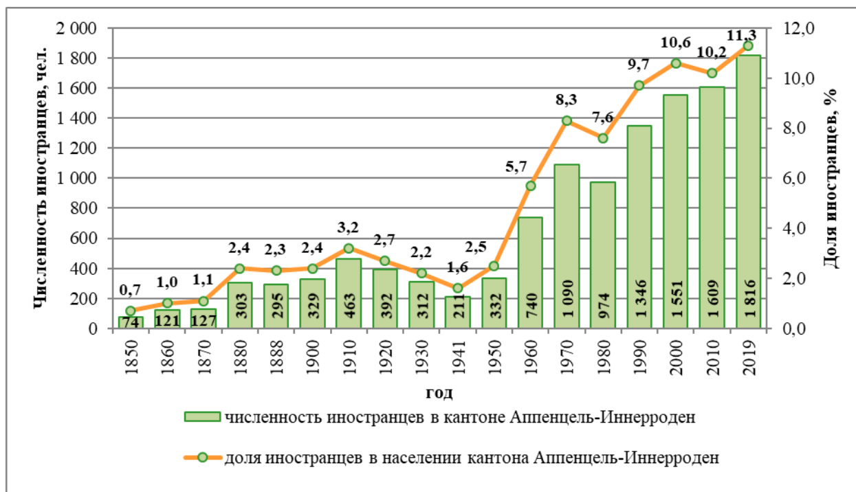
Рис. 17. Численность и доля иностранных граждан в населении кантона Аппенцель-Иннерроден, 1850–2019 гг.
