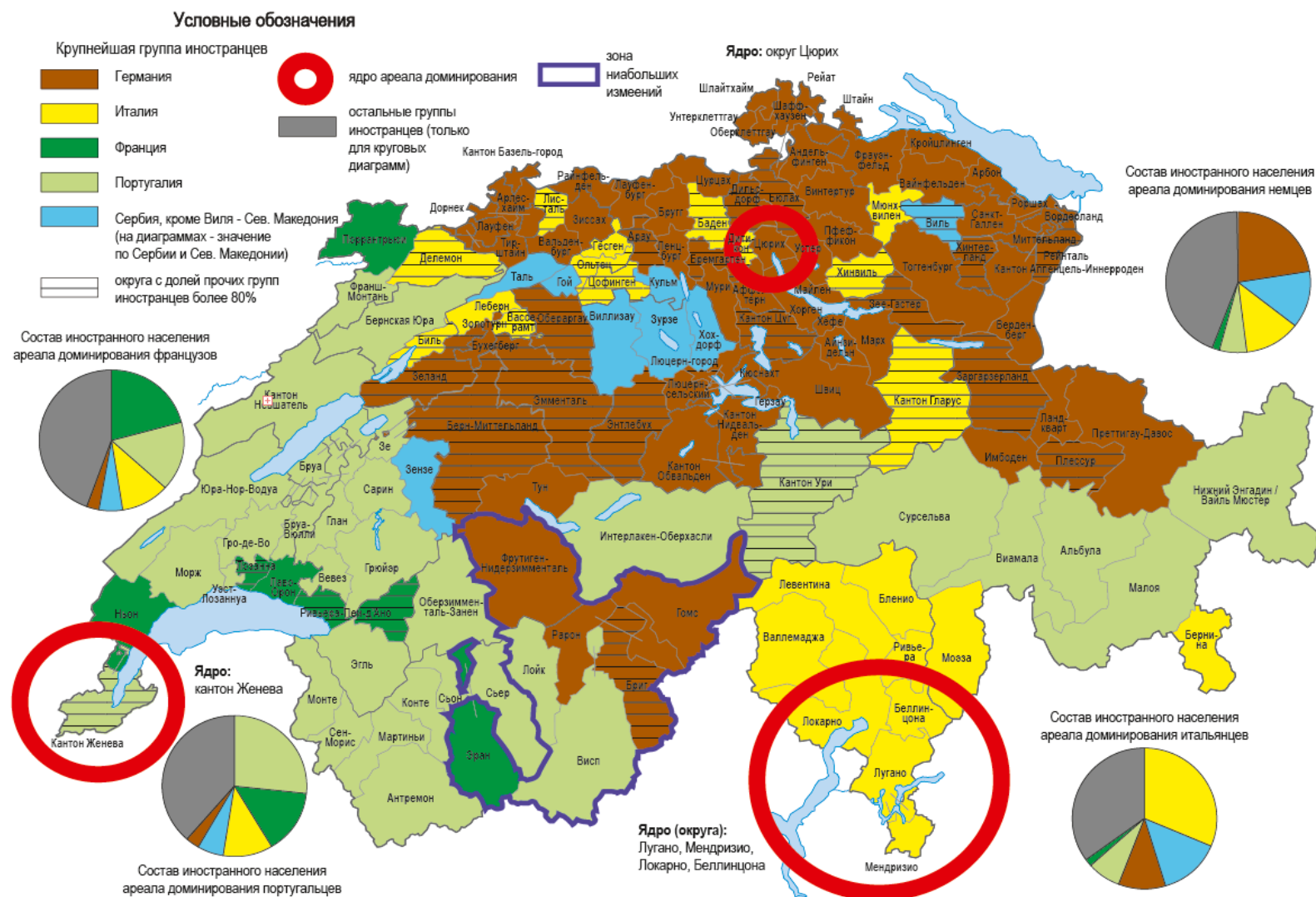
Рис. 20. Ареалы доминирования по округам Швейцарии в 2018 г.
