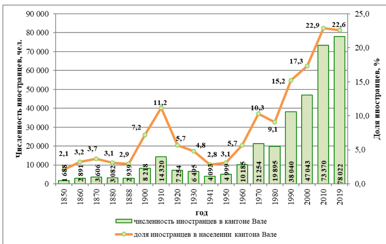
Рис. 7.5. Численность и доля иностранных граждан в населении кантона Вале, 1850–2019 гг.
