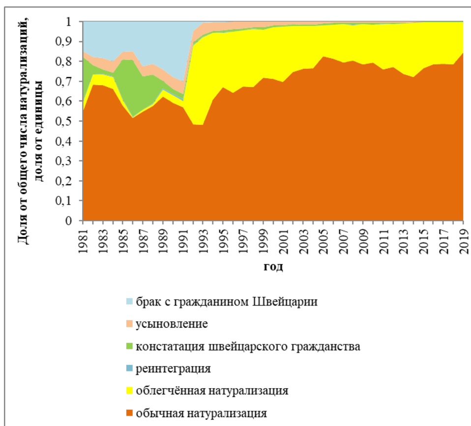
Рис. 3. Получение швейцарского гражданства по способу, 1981–2019 гг.
