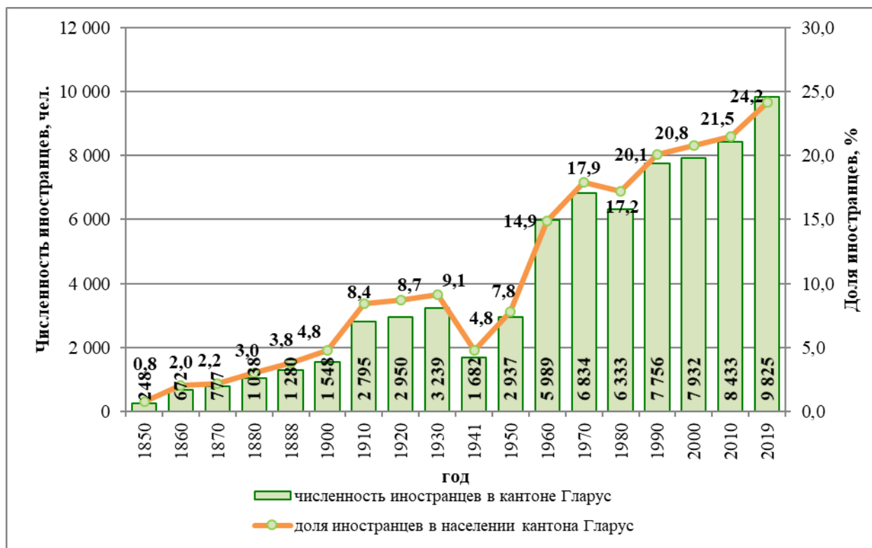
Рис. 15. Численность и доля иностранных граждан в населении кантона Гларус, 1850–2019 гг.
