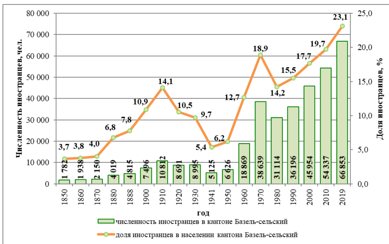
Рис. 7.3. Численность и доля иностранных граждан в населении кантона Базель-сельский, 1850–2019 гг.
