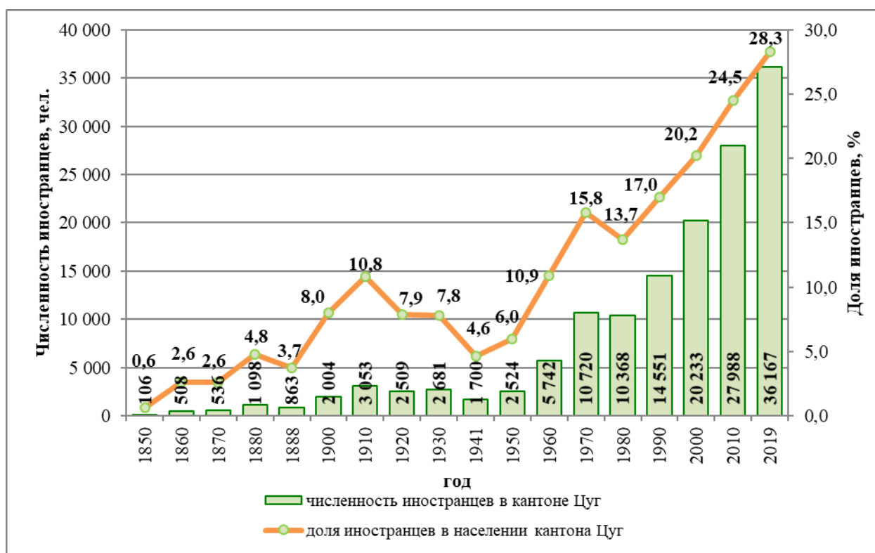
Рис. 7.16. Численность и доля иностранных граждан в населении кантона Цуг, 1850–2019 гг.
