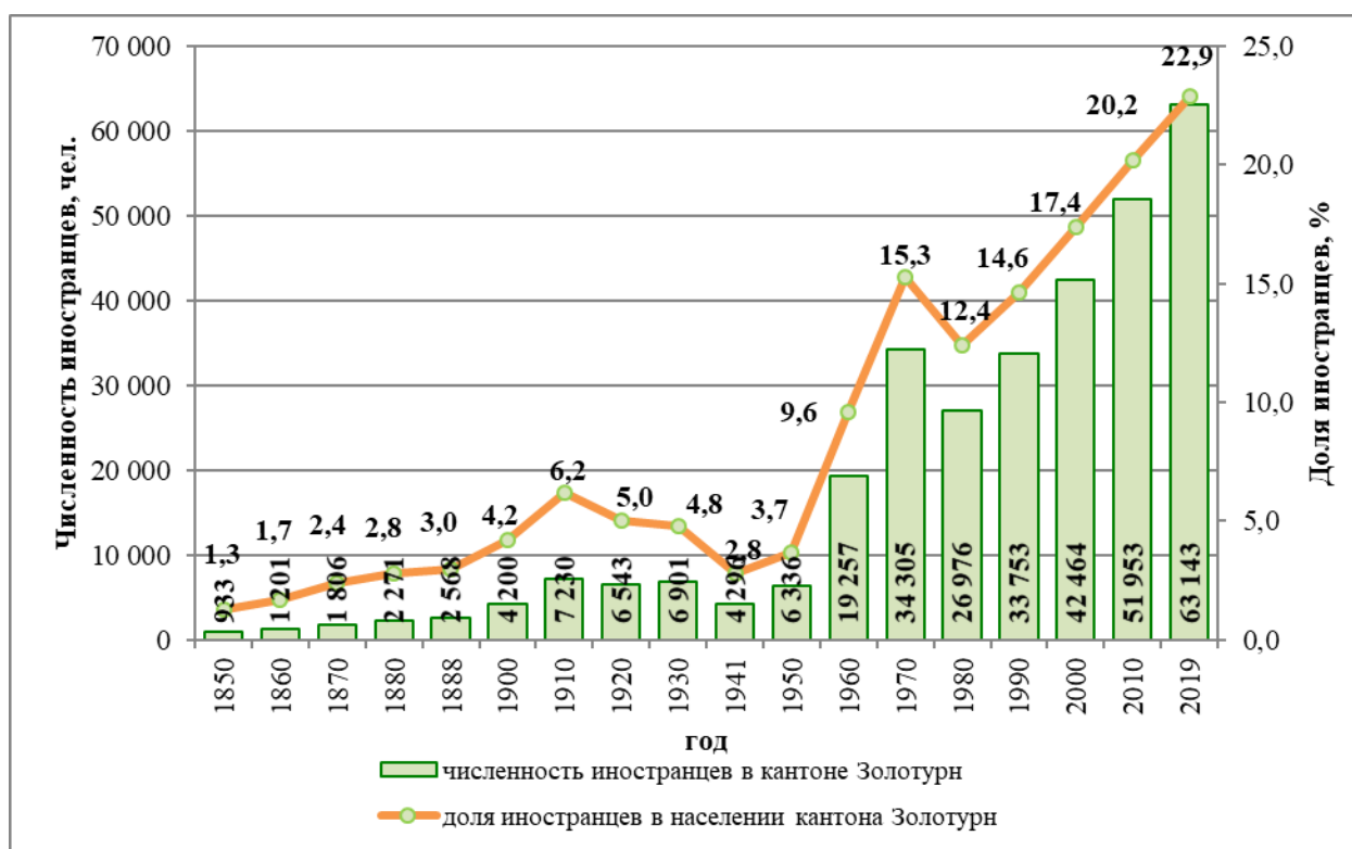
Рис. 7.8. Численность и доля иностранных граждан в населении кантона Золотурн, 1850–2019 гг.
