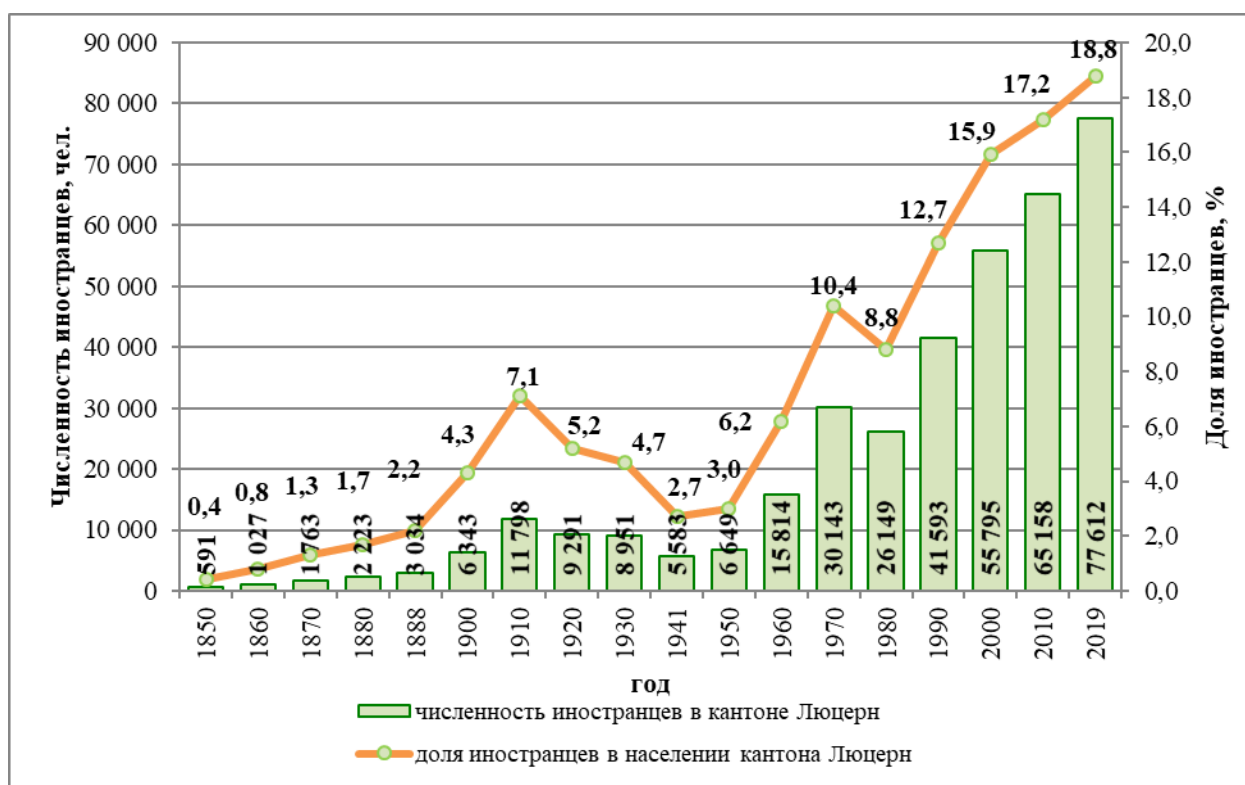
Рис. 7.9. Численность и доля иностранных граждан в населении кантона Люцерн, 1850–2019 гг.
