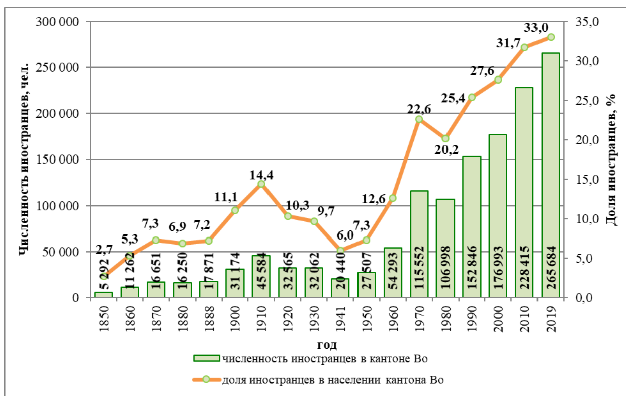
Рис. 7.6. Численность и доля иностранных граждан в населении кантона Во, 1850–2019 гг.
