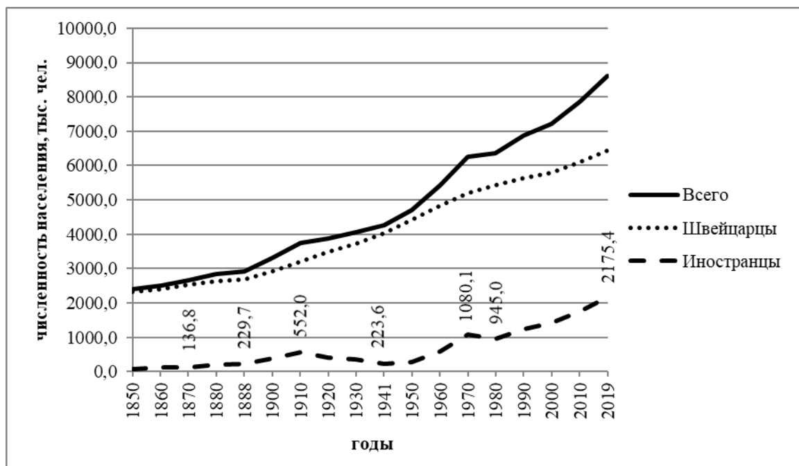
Рис. 10. Динамика численности населения Швейцарии (1850–2019 гг.).
