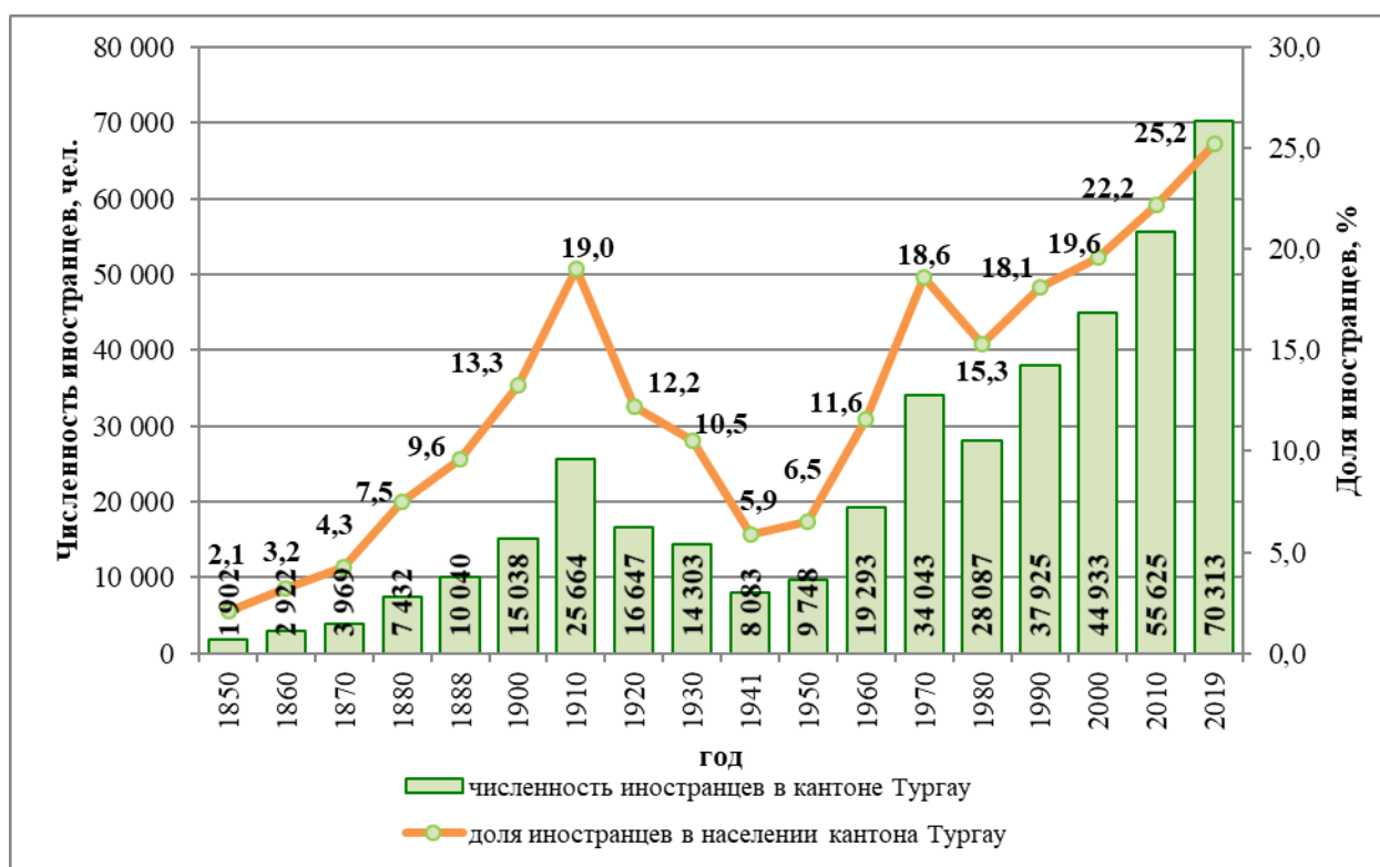
Рис. 7.14. Численность и доля иностранных граждан в населении кантона Тургау, 1850–2019 гг.
