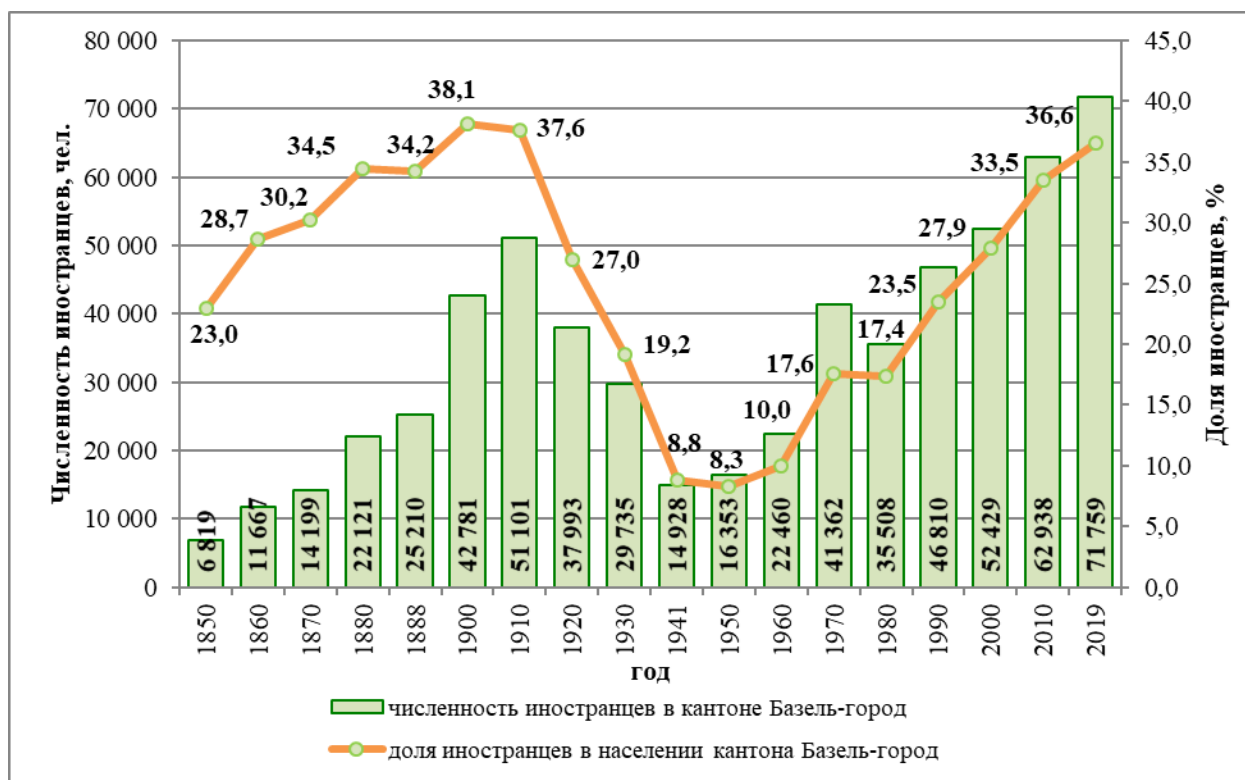
Рис. 13. Численность и доля иностранных граждан в населении кантона Базель-город, 1850–2019 гг.
