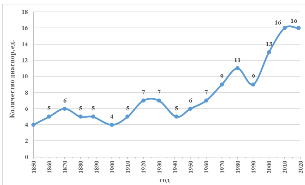
Рис. 5. Количество крупнейших диаспор в Швейцарии, 1850–2019 гг.
