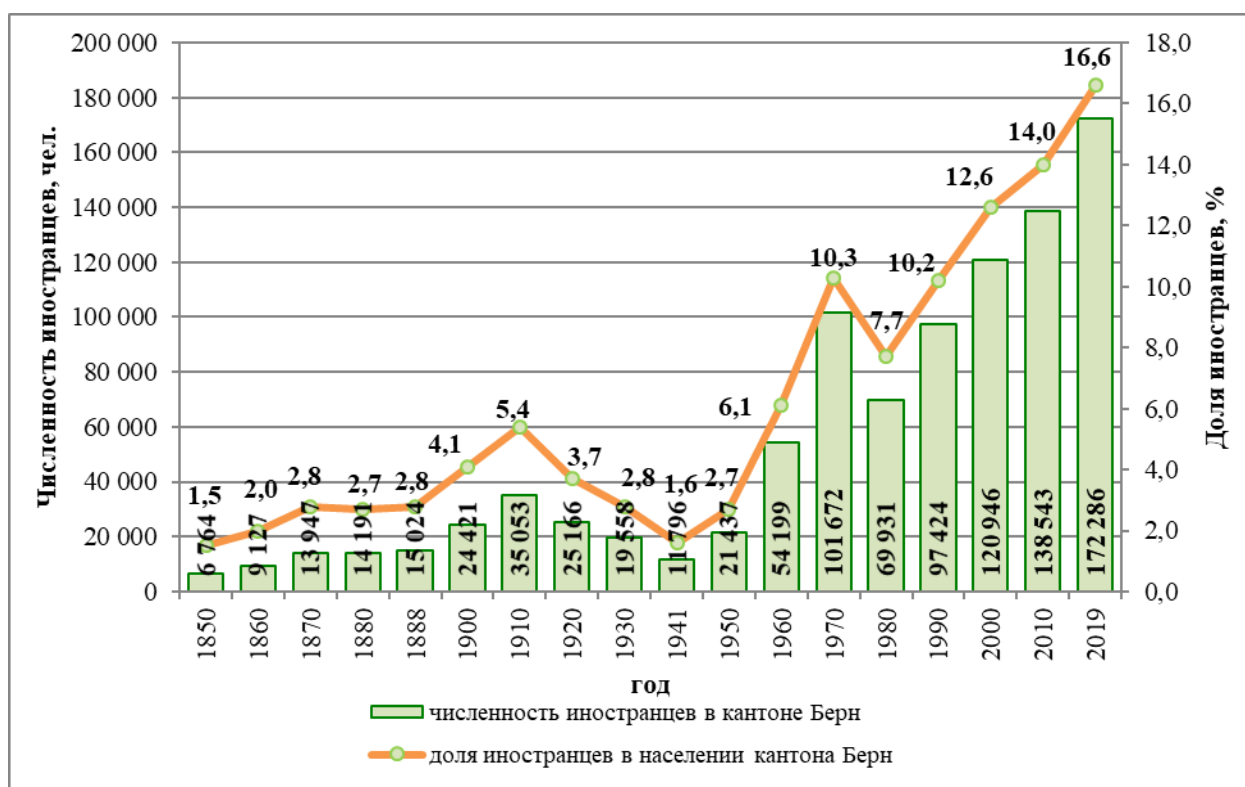
Рис. 7.4. Численность и доля иностранных граждан в населении кантона Берн, 1850–2019 гг.
