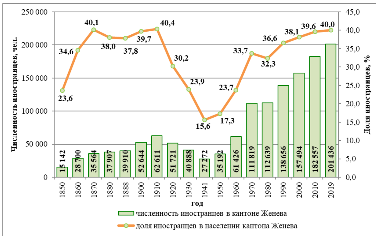
Рис. 12. Численность и доля иностранных граждан в населении кантона Женева, 1850–2019 гг.
