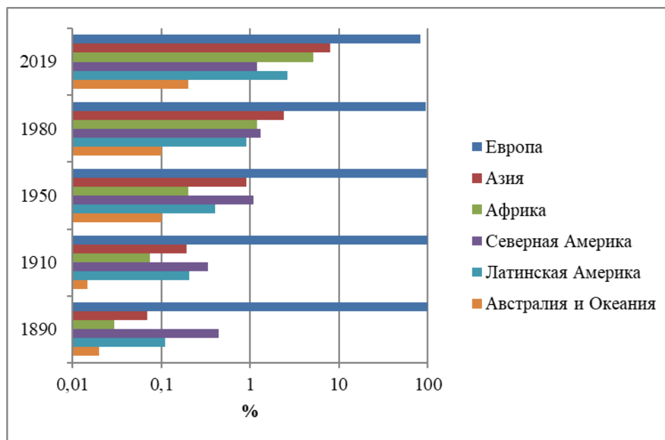
Рис. 4. Доля выходцев из различных макрорегионов мира в иностранном населении Швейцарии
