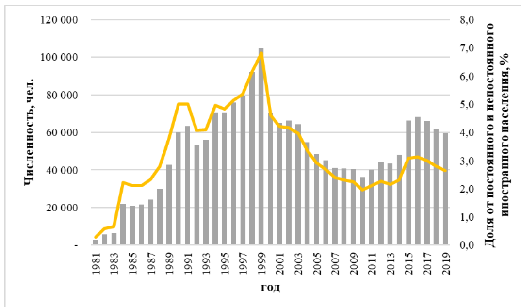
Рис. 2. Численность и доля лиц, ищущих убежище, проживающих (постоянно и непостоянно) на территории Швейцарии, 1981–2019 гг.
