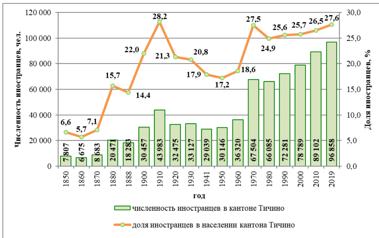
Рис. 14. Численность и доля иностранных граждан в населении кантона Тичино, 1850–2019 гг.
