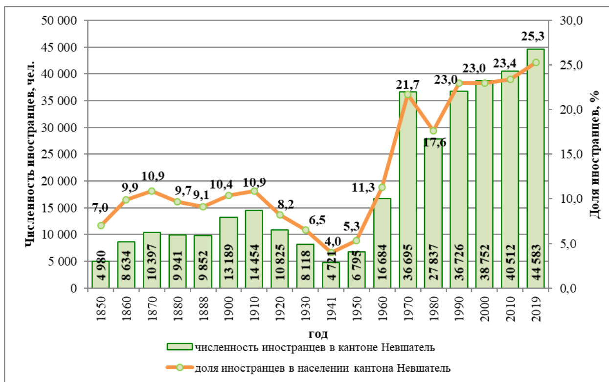
Рис. 7.11. Численность и доля иностранных граждан в населении кантона Невшатель, 1850–2019 гг.
