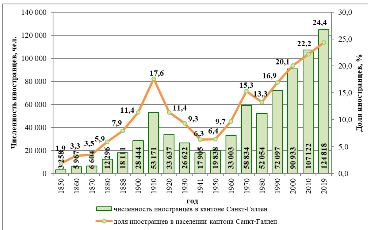
Рис. 7.13. Численность и доля иностранных граждан в населении кантона Санкт-Галлен, 1850–2019 гг.
