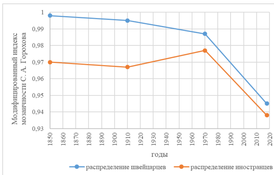
Рис.18. Значения модифицированного индекса мозаичности С. А. Горохова
