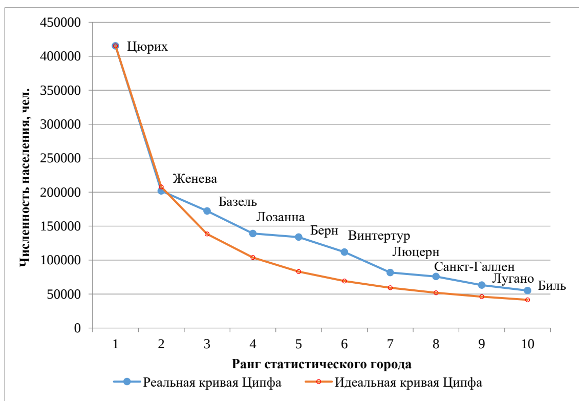
Рис. 21. Распределение крупнейших городов Швейцарии по правилу Ципфа, 2018 год 99
