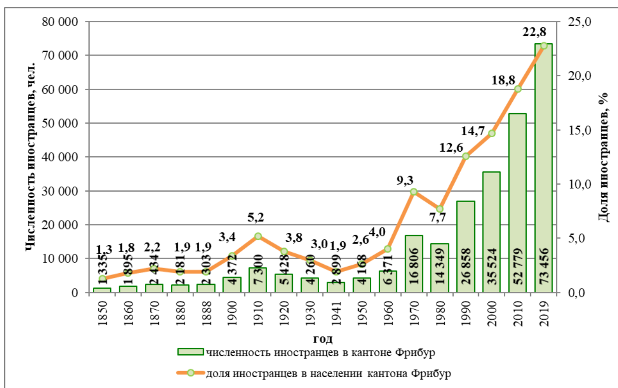
Рис. 7.15. Численность и доля иностранных граждан в населении кантона Фрибур, 1850–2019 гг.
