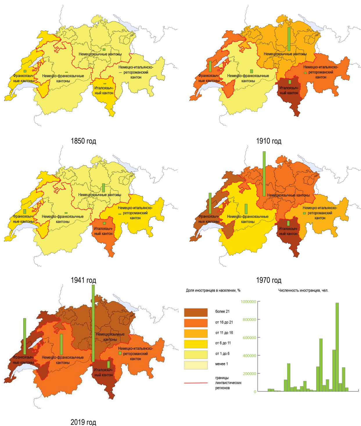
Рис. 11. Численность и доля иностранных граждан, проживающих в лингвистических регионах Швейцарии
