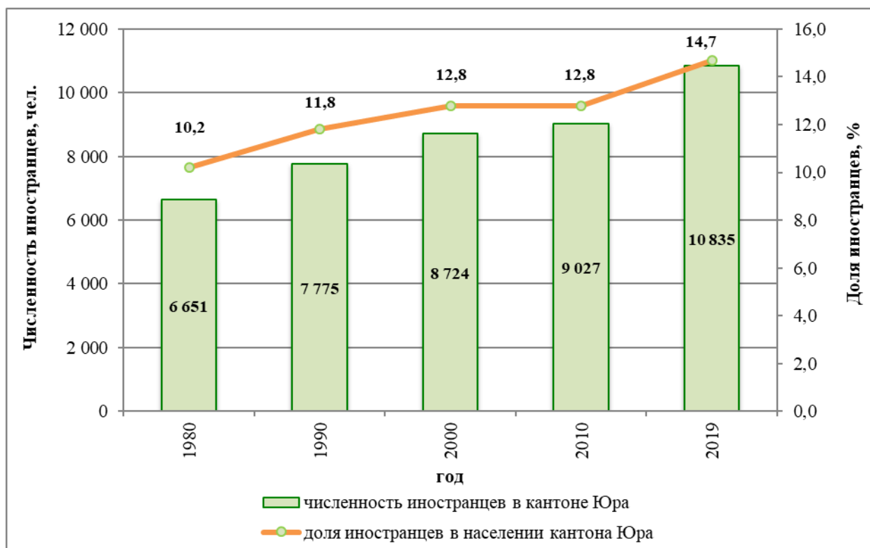
Рис. 7.20. Численность и доля иностранных граждан в населении кантона Юра, 1980–2019 гг.
