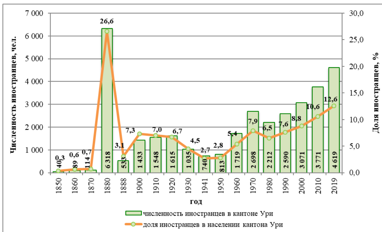
Рис. 16. Численность и доля иностранных граждан в населении кантона Ури, 1850–2019 гг.
