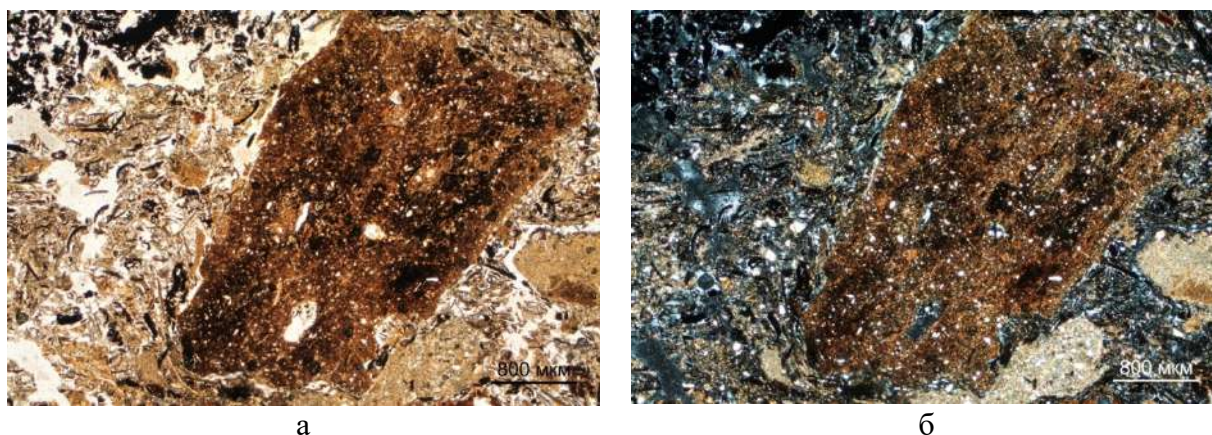
Рис. 59. Фрагмент керамики: железисто-глинистое тонкодисперсное вещества и песчаный грубодисперсный материал. Слой XVIII: а – PPL; б – XPL.
