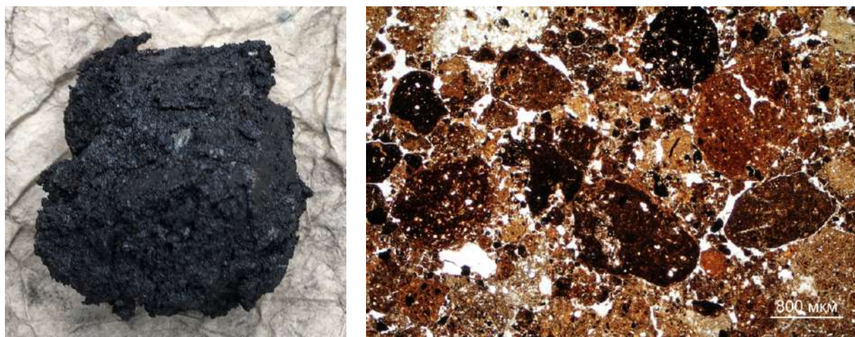
Рис. 10. Слой XI: а – гумусированный суглинок; б – крупные железисто-глинистые агрегаты с глинистыми кутанами вокруг (PPL).
