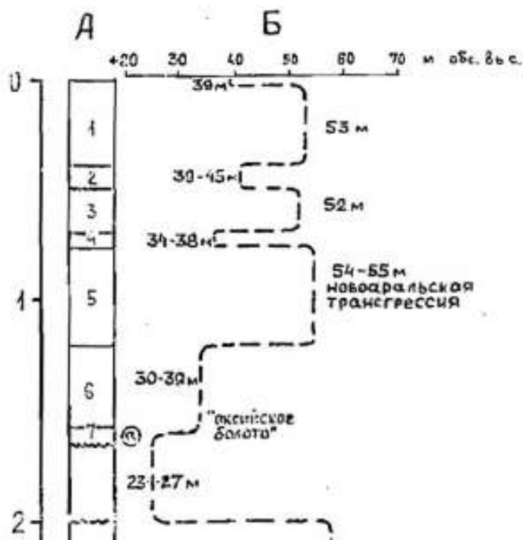
Рис. 40. Уровень Аральского моря за последние 2 тысячи лет. А – временные интервалы накопления слоев донных отложений; Б – положение уровня моря в регрессивные и трансгрессивные эпохи; а – 1500±140 лет (МГУ-778).
