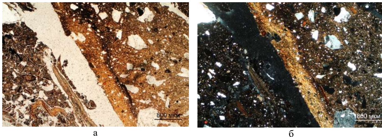
Рис. 27. Фрагмент керамики: железисто-глинистое тонкодисперсное вещество с включением песчано-пылеватых силикатных зерен. Слой XXII: а – PPL; б – XPL.
