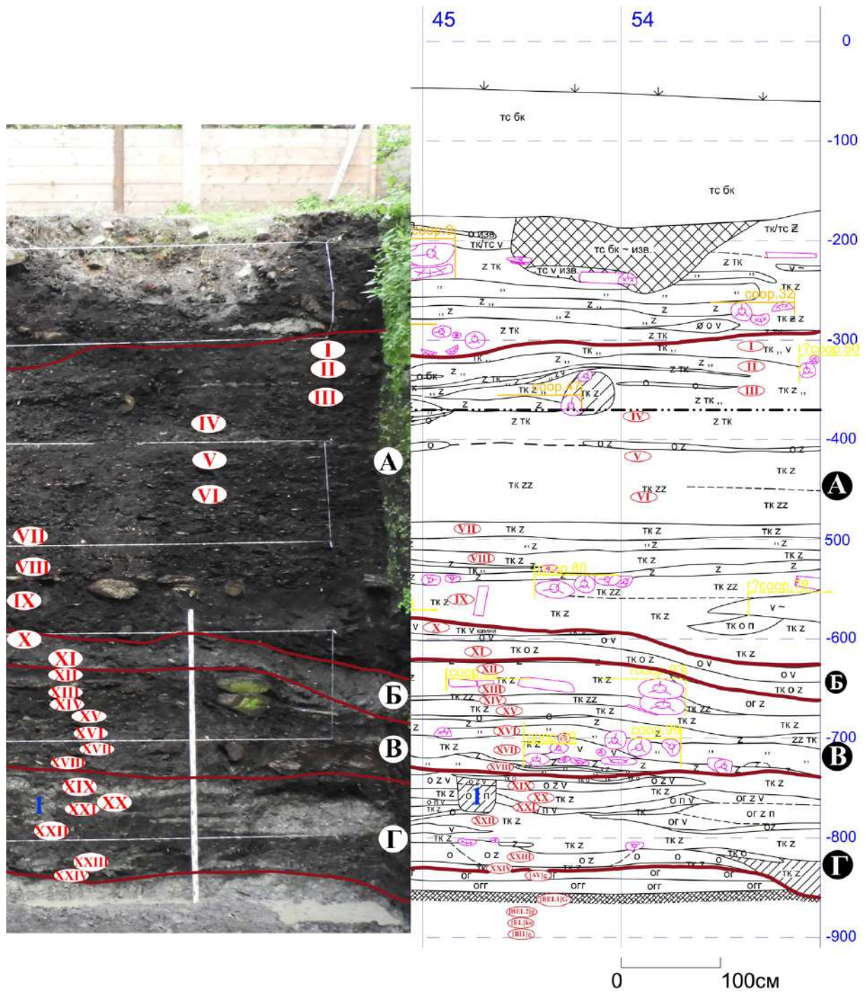
Рис. 7. Стратиграфическое разделение исследуемого профиля на пачки слоев на фотографии (слева) и на чертеже (справа): А – верхняя пачка (слои I-IX), Б – пачка слоев X и XI, В – средняя пачка (слои XII-XVIII), Г – нижняя пачка (слои XIX-XXIV), 1 – яма. Глубины даны в сантиметрах от локального репера.
