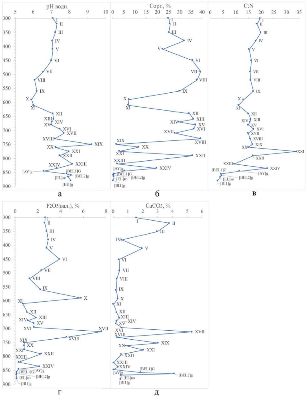
Рис. 19. Данные аналитических исследований стратиграфических слоев: а – рН водн.; б – Сорг, %; в – C:N; г – P 2 O 5 (вал.); д – CaCO 3 , %.
